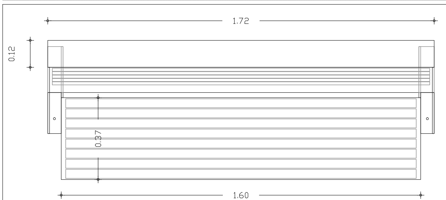
ΚΑΘΙΣΤΙΚΟ ΣΩΜΑ ΜΕ ΠΛΑΤΗ ΠΑΡΑΛΙΑΚΗΣ ΖΩΝΗΣ _ΚΑΤΟΨΗ_ κλίμακα 1/10
